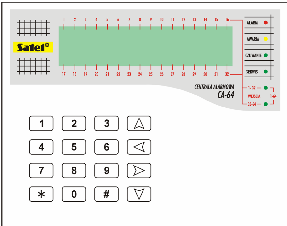
Rysunek 1. Widok manipulatora CA-64 K
