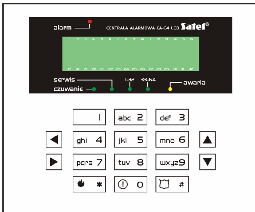
Rysunek 2. Widok manipulatora CA-64 KLCD-S
