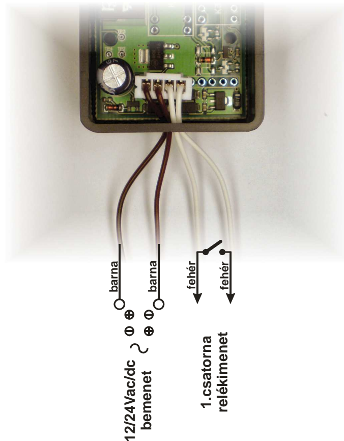
2. ábra: Csatlakozó vezetékek bekötése
