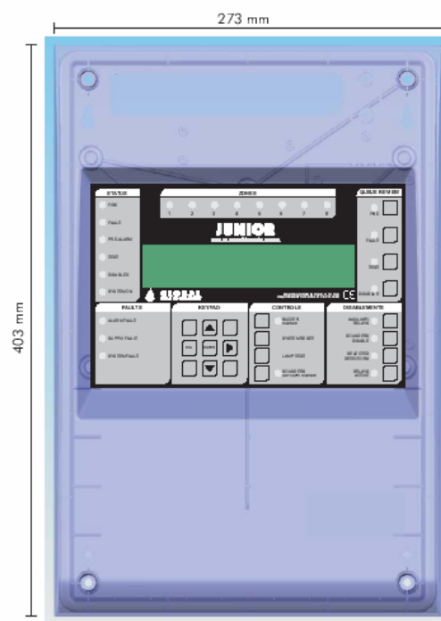
ELŐLNÉZET
