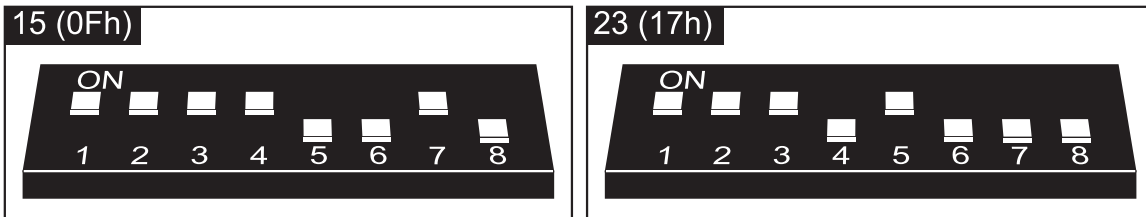
2. Ábra DIP-kapcsolók beállításának példája. A 23 (17h) cím beállítása szükséges VERSA vezérlőpanellel történő használat esetében.
