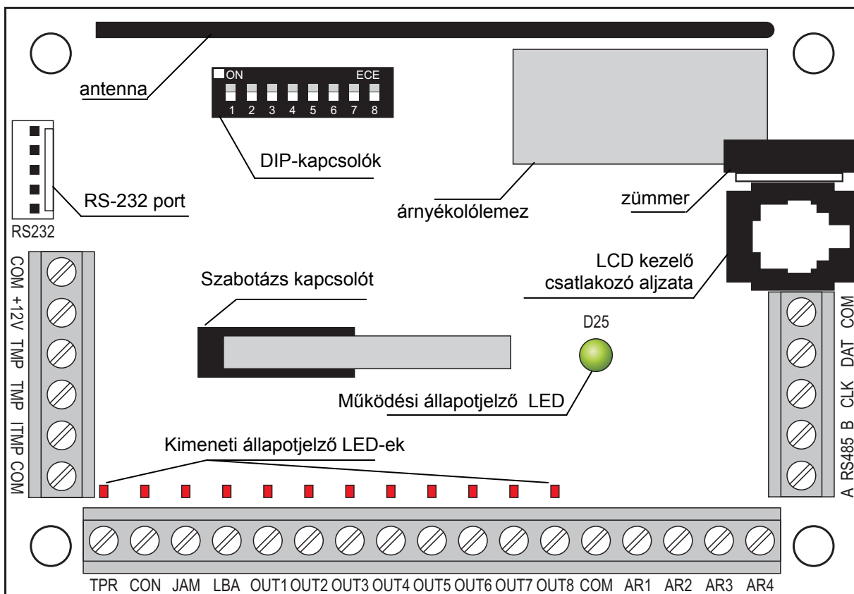
1. Ábra. Az ACU-1000 vezérlő áramköri lapjának vázlatos nézete.
