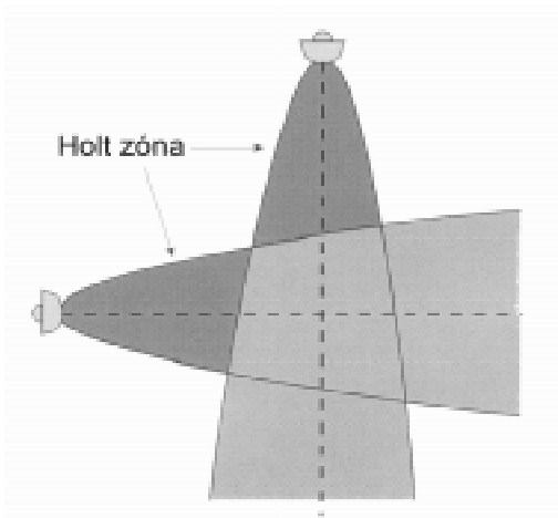
21b ábra - Két érzékenységi sáv átfedése egy metszéspontban
