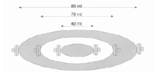
2. ábra - Az érzékeny zóna méretének változása a távolság változásának függvényében
