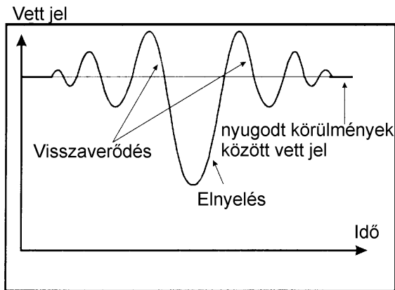
7. ábra - A behatolás alatt kapott jel reprezentációja
