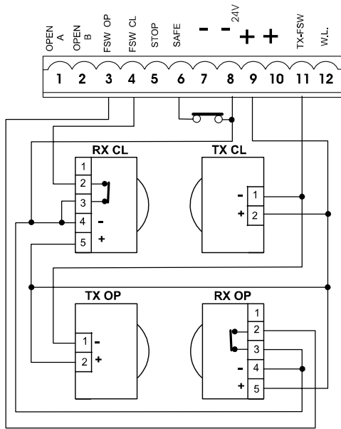
Aansluiting van een paar fotocellen bij opening, een paar bij sluiting en een veiligheidslijst
