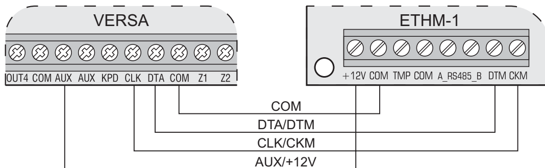
12. Ábra ETHM-1 modul csatlakoztatásának módja. Ha a vezérlőpanel Ethernet hálózaton keresztül távolról van programozva szükséges továbbá az ETHM-1 modul RS-232 portjának (PIN-5 típusú aljzat) csatlakoztatása a panel RS-232 portjához egy SATEL gyármánú PIN5/RJ-TTL kábel használatával.
