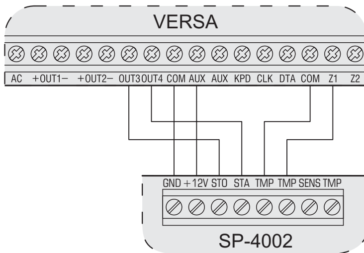
28. ábra Saját tápellátással rendelkező sziréna csatlakoztatása a vezérlőpanelre (például SP-4002). Az OUT3 és OUT4 kimenetek ellentétes polaritású programozása szükséges. A sziréna PLA és PLO érintkező tűskéit rövidre kell zárni (riasztásindítás, ha közös föld megszűnik).
