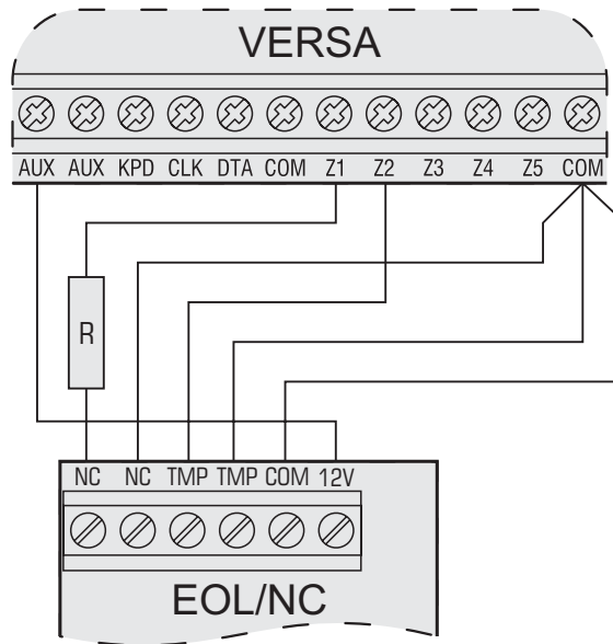
25. ábra Példa NC típusú érzékelők központhoz csatlakoztatására EOL konfigurációban.
