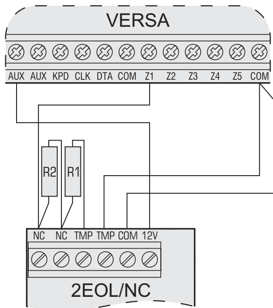
26. ábra Példa NC típusú érzékelők központhoz csatlakoztatására 2EOL konfigurációban (NO típusú érzékelők csatlakoztatása ugyanígy történik).
