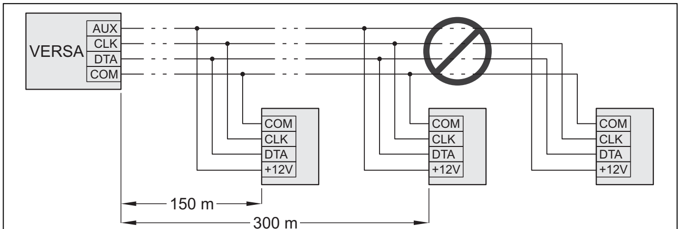
5. ábra Saját tápellátással nem rendelkező modulok csatlakoztatása, ha távolság a központ és a modul között nem haladja meg a 300 métert. A modulok tápellátása a központról történik. Egy-egy 0.5 \text{ mm}^2 keresztmetszetű vezeték használható az egyes jeleknek (CLK, DTA, COM). 300 méternél nagyobb távolságú modulok csatlakoztatása ilyen módon nem lehetséges.
