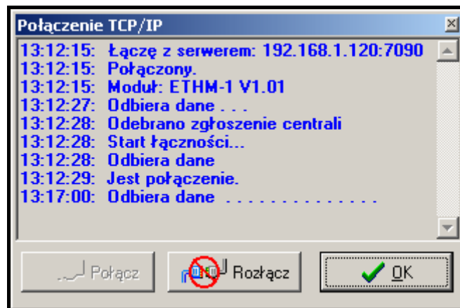
Rys. 5. Okno „Połączenie TCP/IP” w programie DLOADX z komunikatami, które pojawiają się w trakcie nawiązywania komunikacji z centralą.
