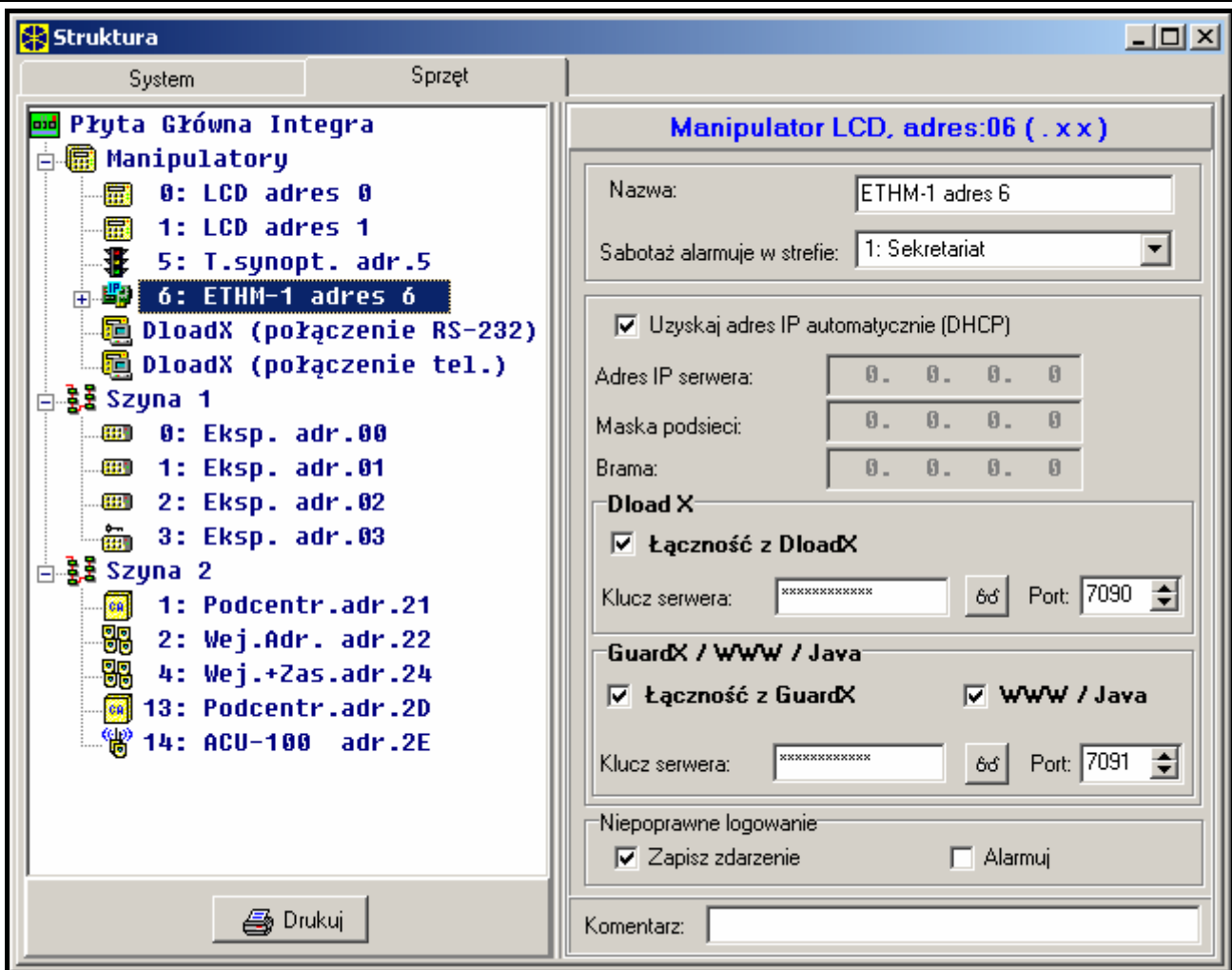
Rys. 3. Okno ustawień modułu ETHM-1 w programie DLOADX.
