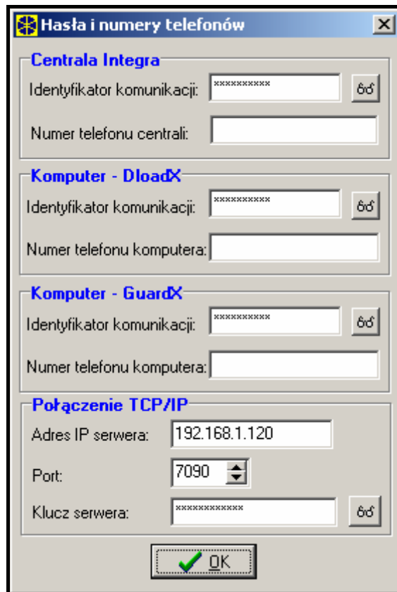
Rys. 4. Okno przykładowych ustawień komunikacji w programie DLOADX.
