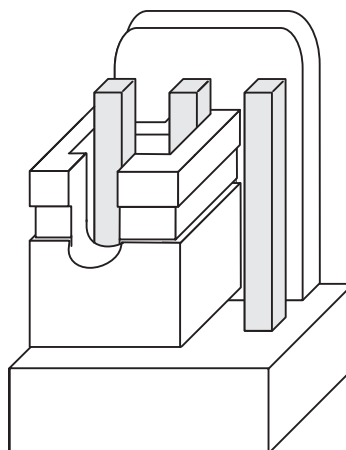
22. ábra Rövidzár felhelyezésének módja az RS-232 TTL port érintkezőire.
