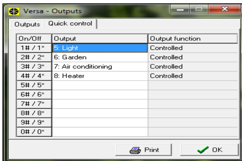
11. ábra. Kimenet hozzárendelése a megfelelő kezelő gombokhoz a DLOADX programban (példa).
