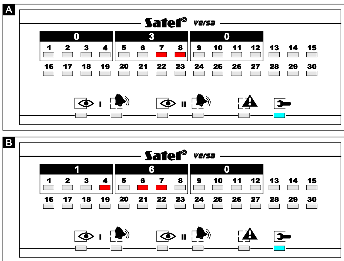
1. ábra. Példa decimális értékek kijelzésére LED-ek használatával LED kezelőn. A 30-as értéket (030) mutatja az „A” példa, a 160-es értéket pedig „B” példa.
