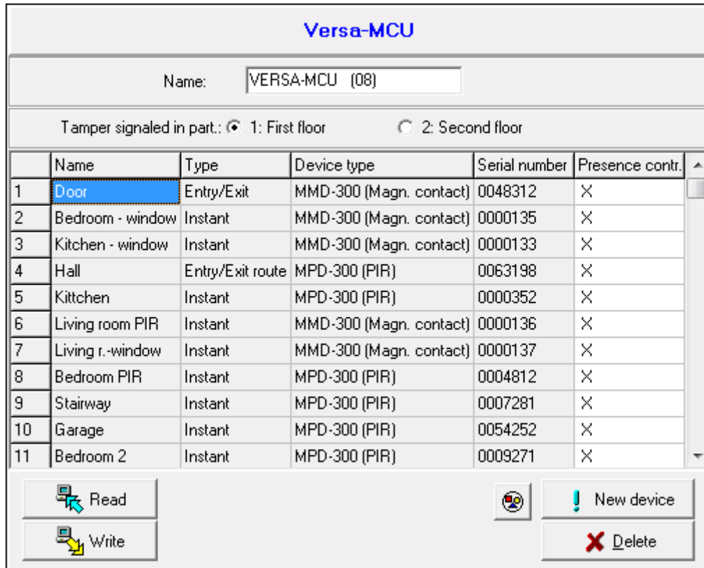
15. ábra 433 MHz vezeték nélküli rémóndszer-vezérlő és 433 MHz érzékelők beállításainak programozása a DLOADX programban (példa).
