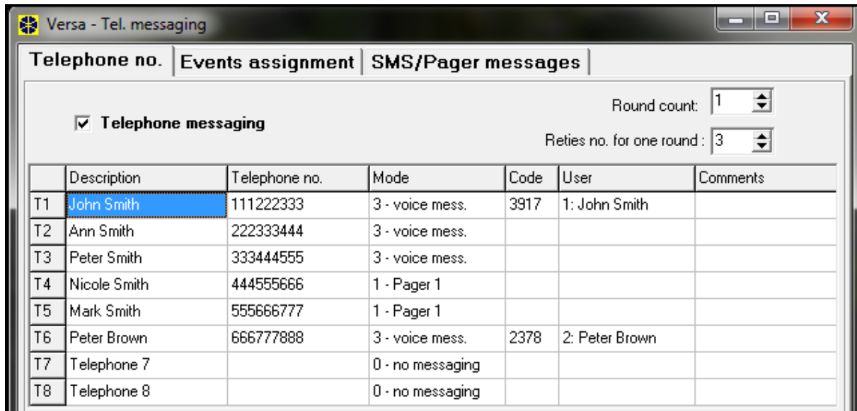
19. ábra Üzenetküldési paraméterek programozása a DLOADX programban (példa konfiguráció).
