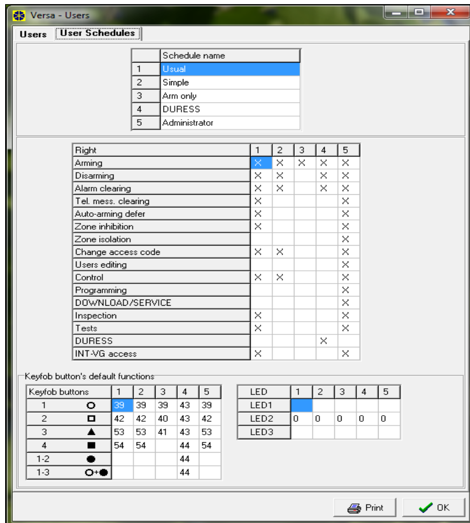
20. ábra. Felhasználó profilok programozása a "Versa – Felhasználók" ablakban, a DLOADX programban (példa konfiguráció).
