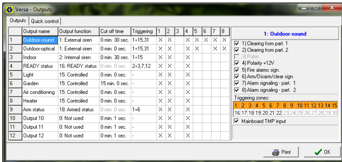
10. ábra "Versa – Kimenetek" ablak a DLOADX programban.
