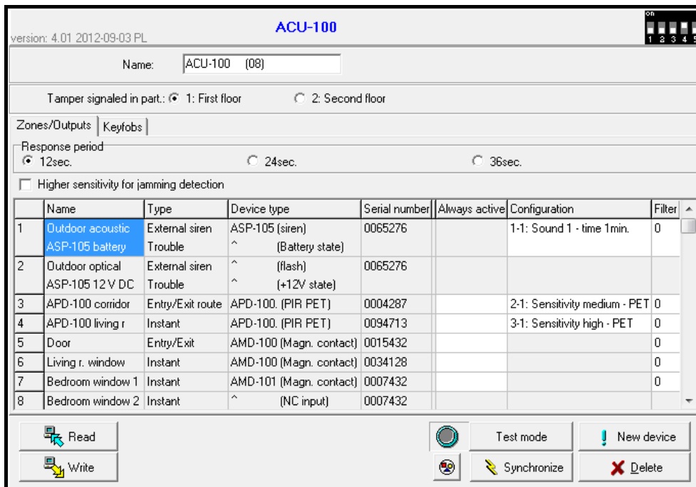
14. ábra. Vezetéknélküli rendszer vezérlő és vezetéknélküli eszközök beállításainak konfigurálása a DLOADX programban (példa konfiguráció).
