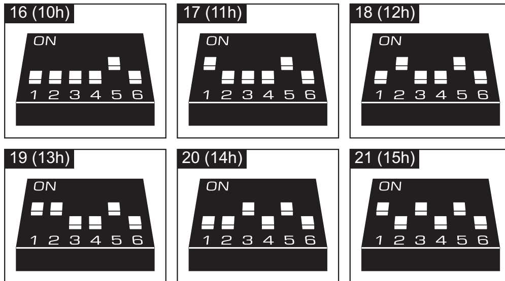
Rys. 21. Sposób ustawienia adresów w czytnikach INT-IT.
