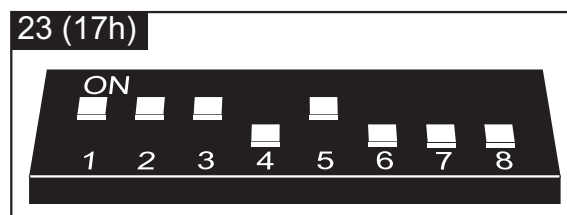
Rys. 22. Sposób ustawienia adresu w syntezerze CA-64 SM. Ósmy przełącznik jest w pozycji OFF, czyli funkcja nagrywania komunikatów głosowych jest zablokowana.
