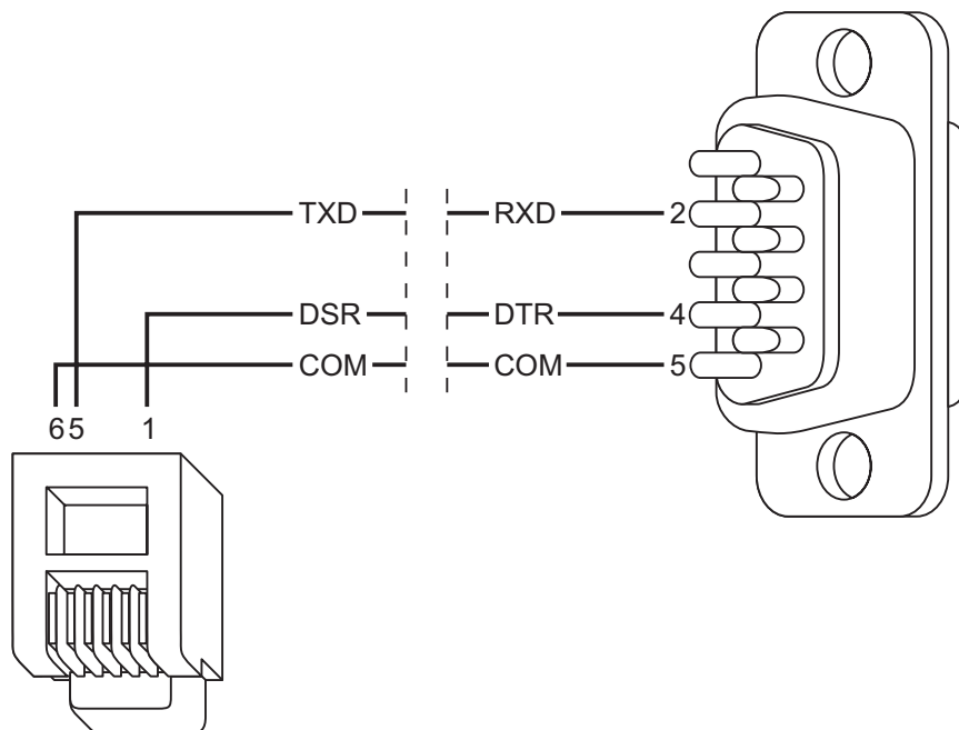
Rys. 24. Sposób podłączenia drukarki przy pomocy wtyku męskiego DB-9 (widok od strony punktów lutowniczych).
