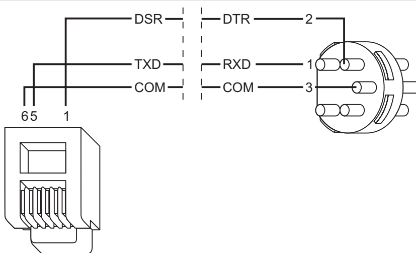
Rys. 25. Sposób podłączenia drukarki przy pomocy 5-pinowego wtyku DIN (widok od strony punktów lutowniczych).
