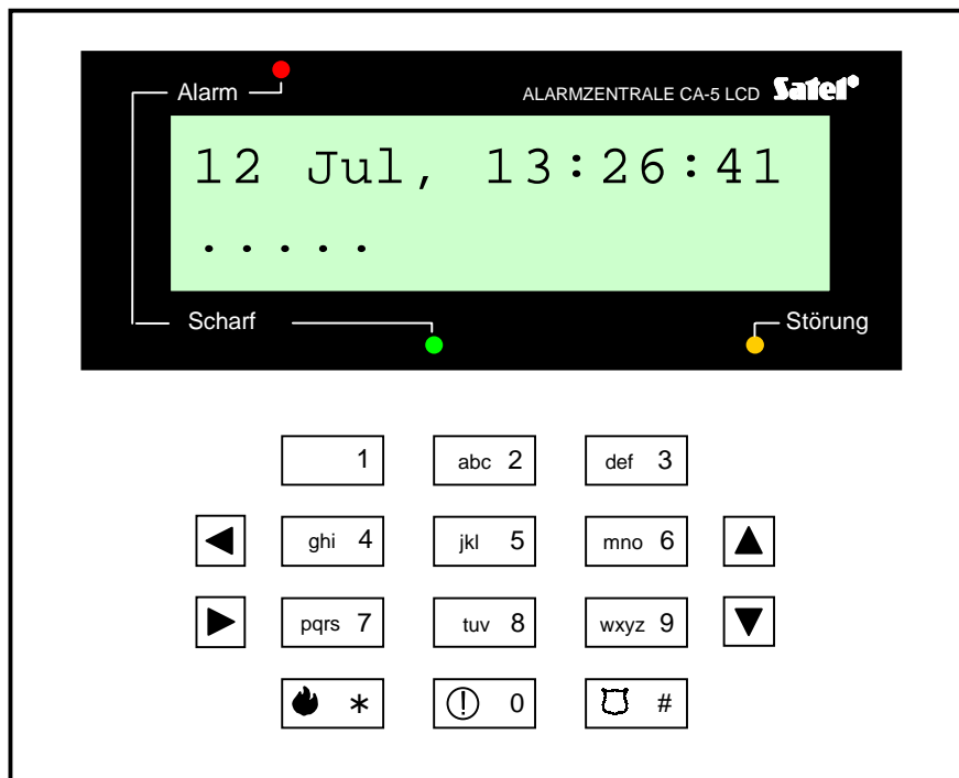
Abbildung 1. Bedienteil LCD-L der Zentrale CA-5.
