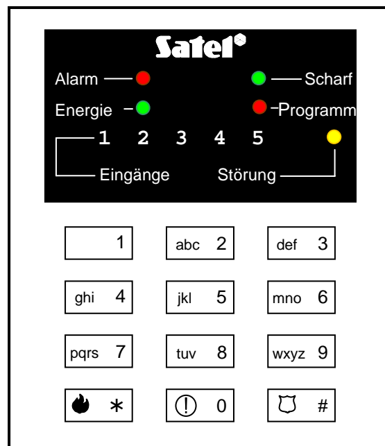
Abbildung 1. Bedienteil CA-5 KLED-S.
