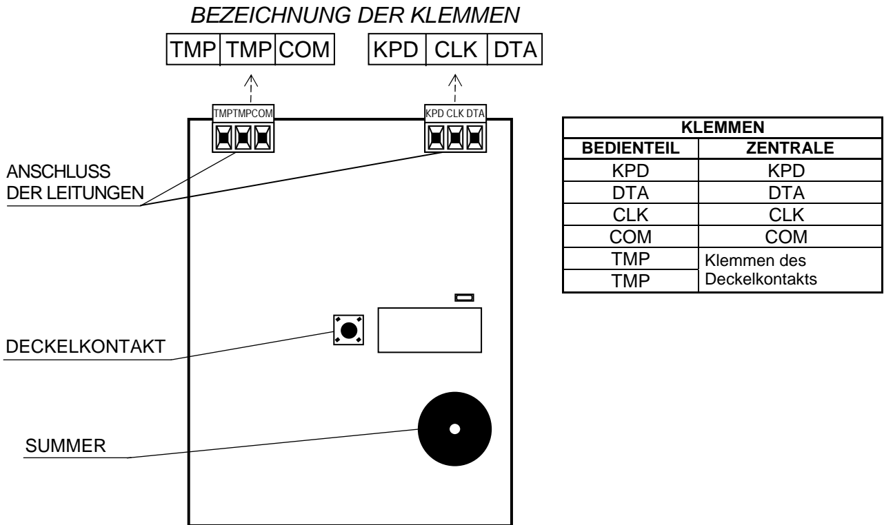
Abbildung 2. – Platine des Bedienteils in der Version CA4/5/8/12/16KN V1.1.
