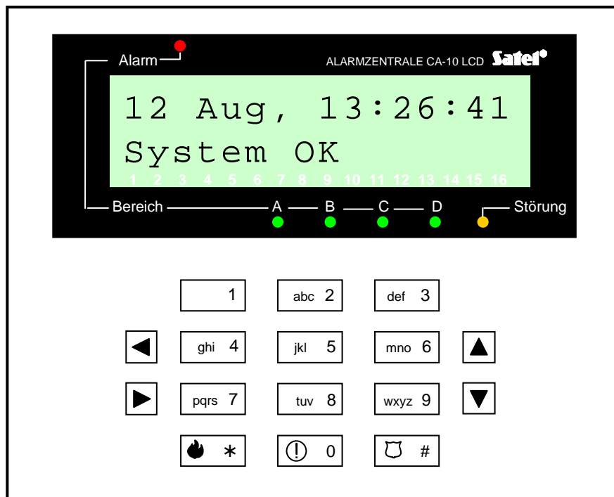
Abbildung 1. Bedienteil LCD-L der Zentrale CA-10.
