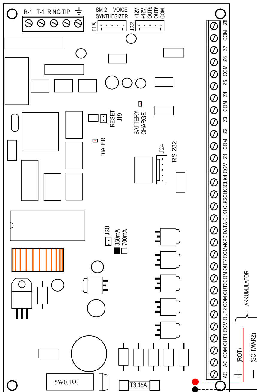
Abb. 1 – Ansicht der Platine in der Ausführung CA10PV4.3.
