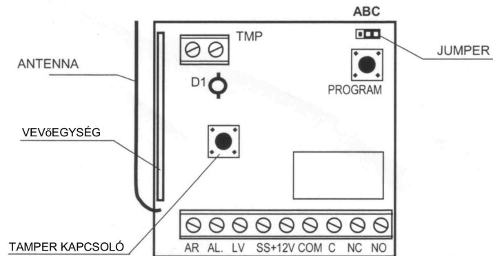
1.ábra: az 1 csatornás kontroller panelje
