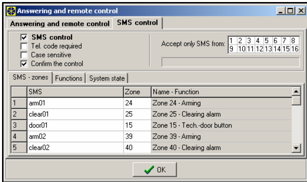
25. ábra SMS vezérlés beállítás
