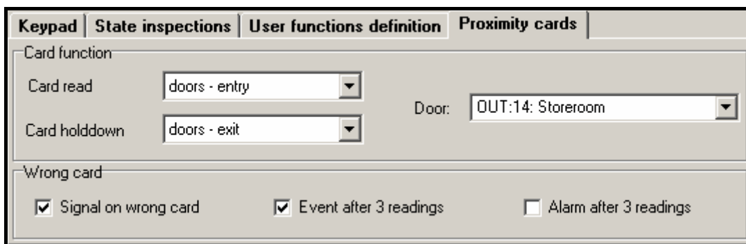
16. ábra Proximitykártyák kezelése.
