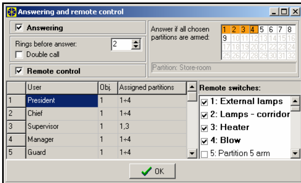
24. ábra Felhasználók által vezérelhető távoli kapcsolók meghatározása.
