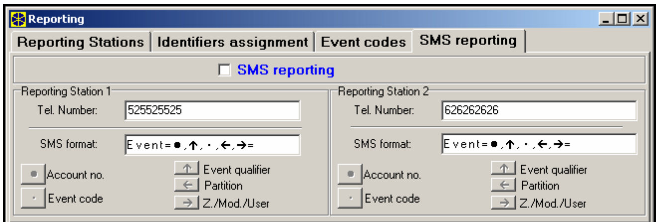
18. ábra „Jelentés” ablak SMS felügyelet beállítás füle.
