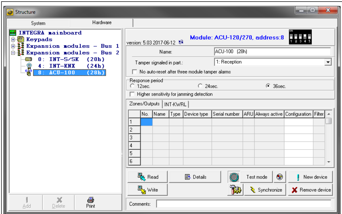
3. ábra DLOADX program: INTEGRA / INTEGRA Plus vezérlőpanelhez csatlakoztatott vezérlő paraméterei és opciói.
