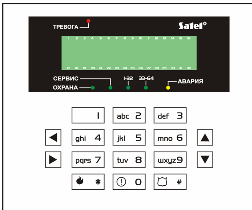
Рис.2. Вид клавиатуры CA-64 KLCD-S
