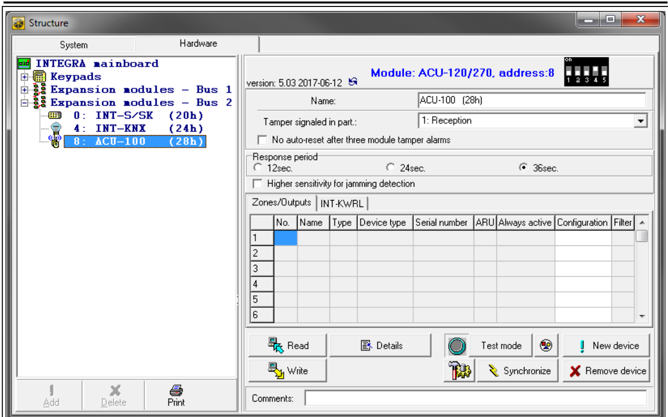
3. ábra DLOADX program: INTEGRA / INTEGRA Plus vezérlőpanelhez csatlakoztatott vezérlő paramétereit és opcióit.
