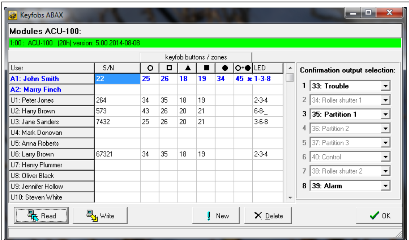
5. ábra DloadX program: távvezérlők kezelése INTEGRA / INTEGRA Plus vezérlőpanelhez csatlakoztatott vezérlő esetén.
