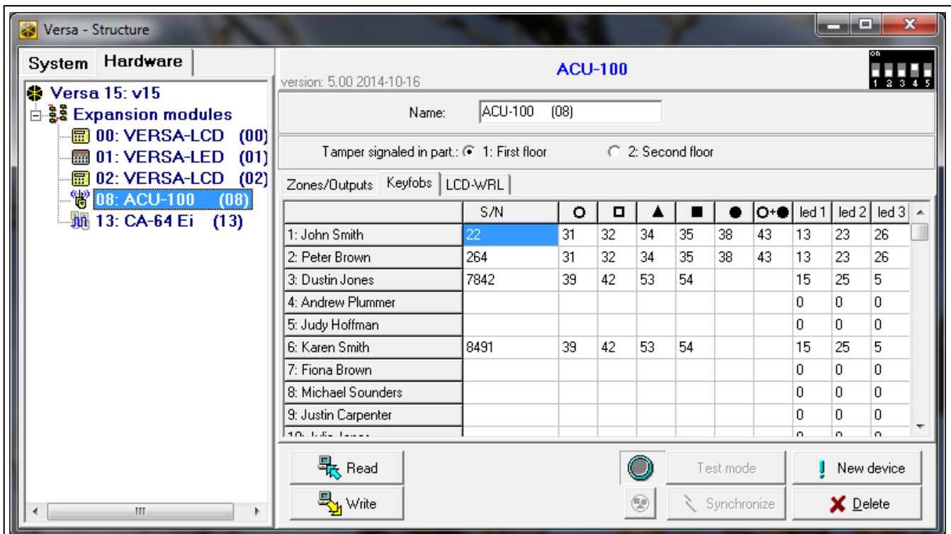
6. ábra DloadX program: távvezérlők kezelése VERSA / VERSA Plus / VERSA IP vezérlőpanelhez csatlakoztatott vezérlő esetén.
