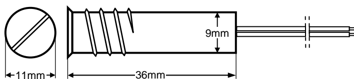
Rys. 3 Kontaktron czujki K-3 w obudowie metalowej
