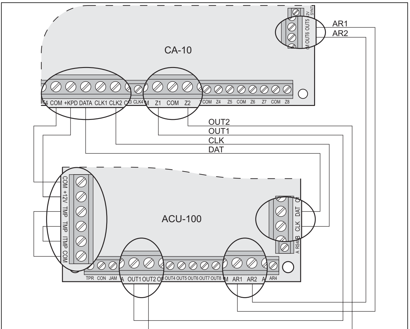
12. Ábra Példa az ACU-100 vezérlő CA-10 riasztóközpontoz történő csatlakoztatására.
