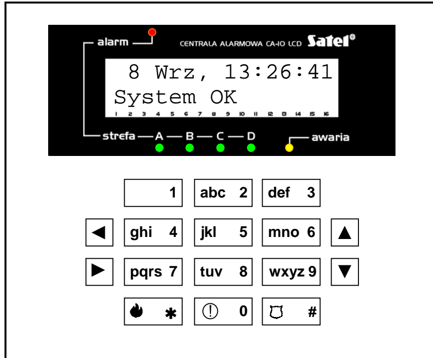
Manipulator typu CA-10 KLCD-S. Manipulatory CA-10 KLCD-S i CA-10 KLCD-L różnią się między sobą wymiarami zewnętrznymi i wielkością wyświetlacza.
