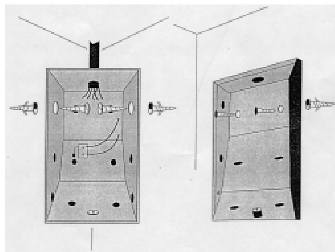
2. ábra – FELSZERELÉS sarokba, vagy falra
