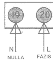
4-ES SORKAPOCS
