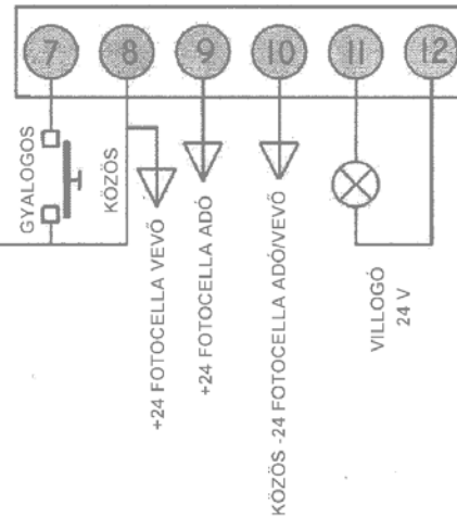
2B SORKAPOCS
