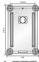
Wall Mount (STB-LM)
