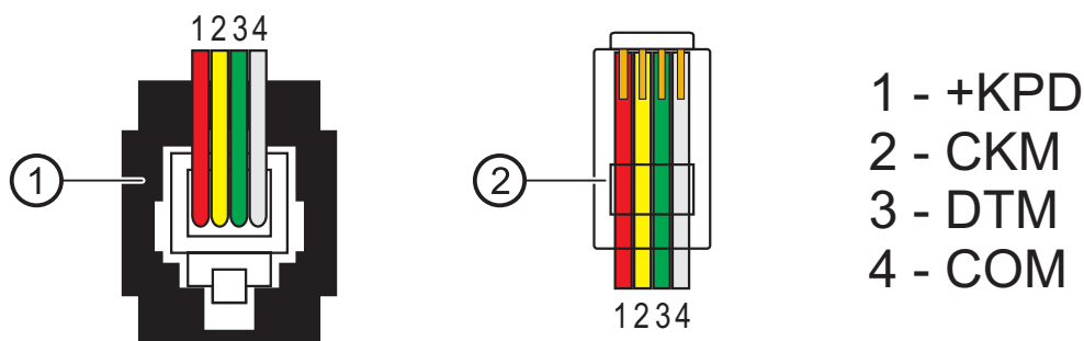
3. ábra A vezérlőhöz csatlakoztatott LCD kezelő vezetékének sorrendje a csatlakozódugóban.
